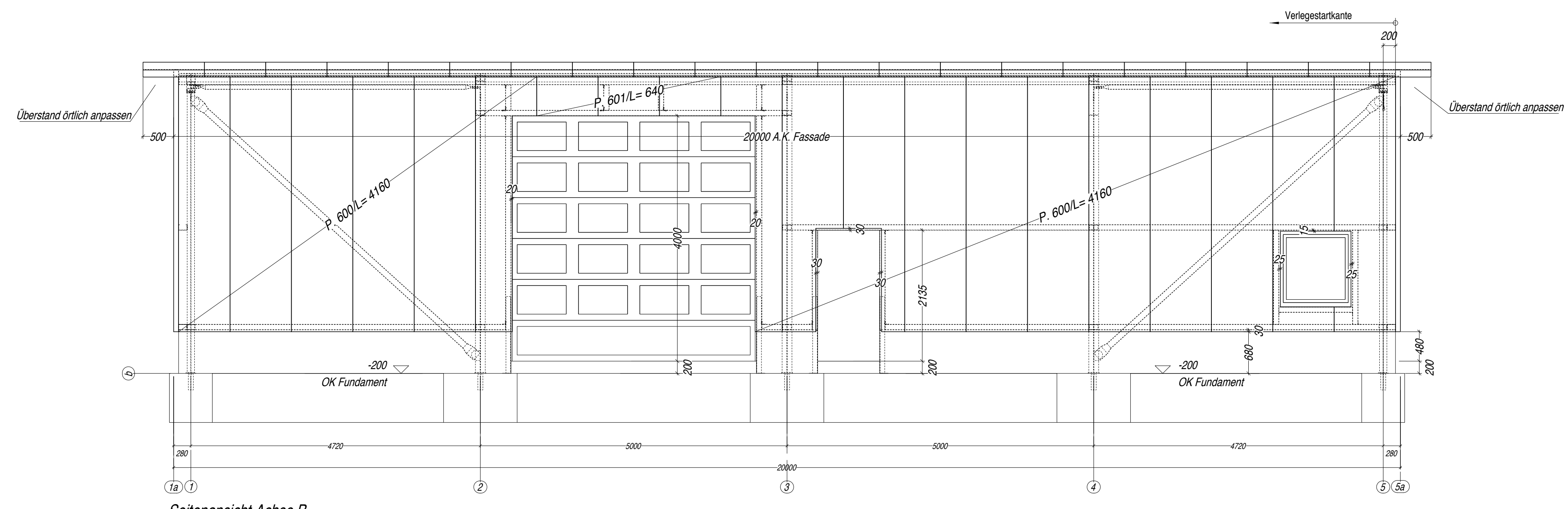
Seitenansicht Achse B Maßstab: 1:50
