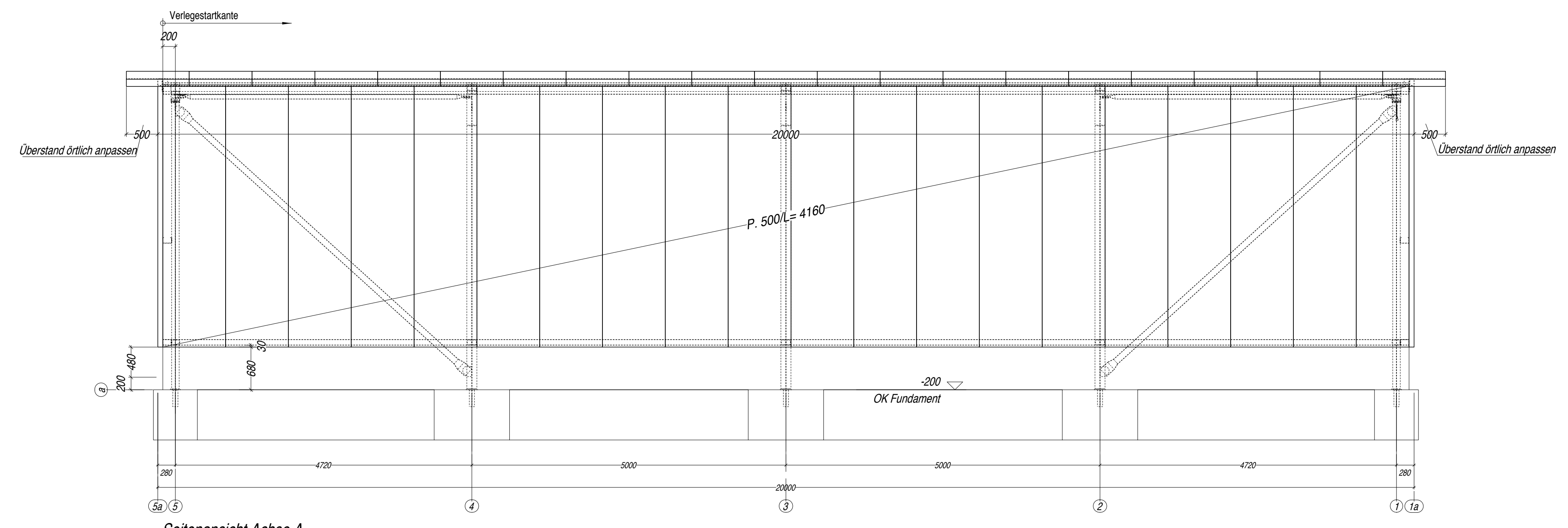
Seitenansicht Achse A Maßstab: 1:50
